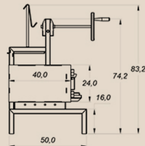
Bison Modelo 3 - 1140x500 - VISTA LATERAL ESQUERDA
