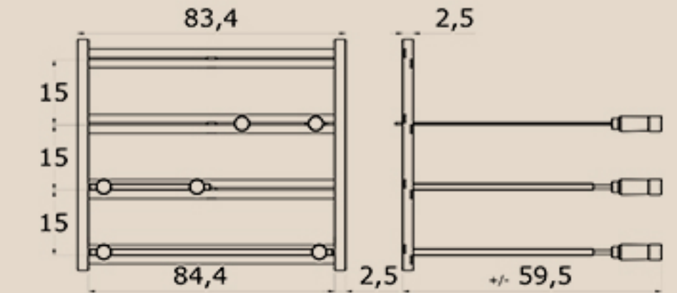
Grill Ossoboca Parede Modelo 4
