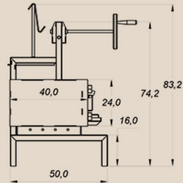
Bison Modelo 1 - 740x500 - VISTA LATERAL ESQUERDA
