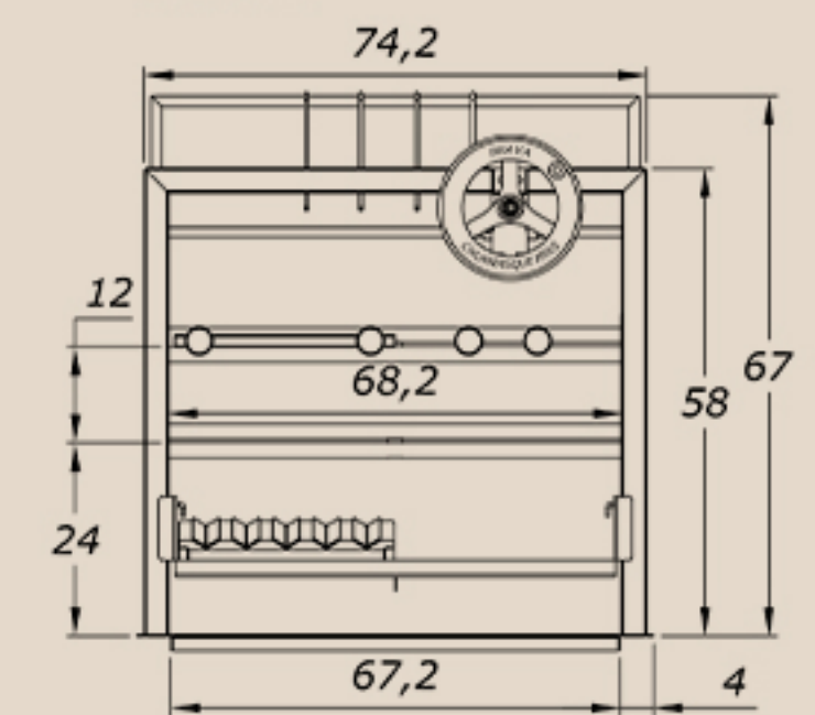
Elevation Grill Modelo 3
