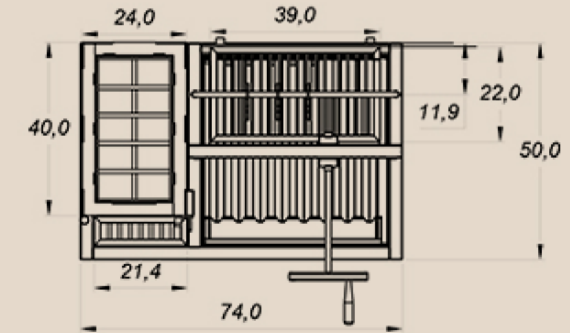
Bison Modelo 1 - 740x500 - VISTA SUPERIOR
