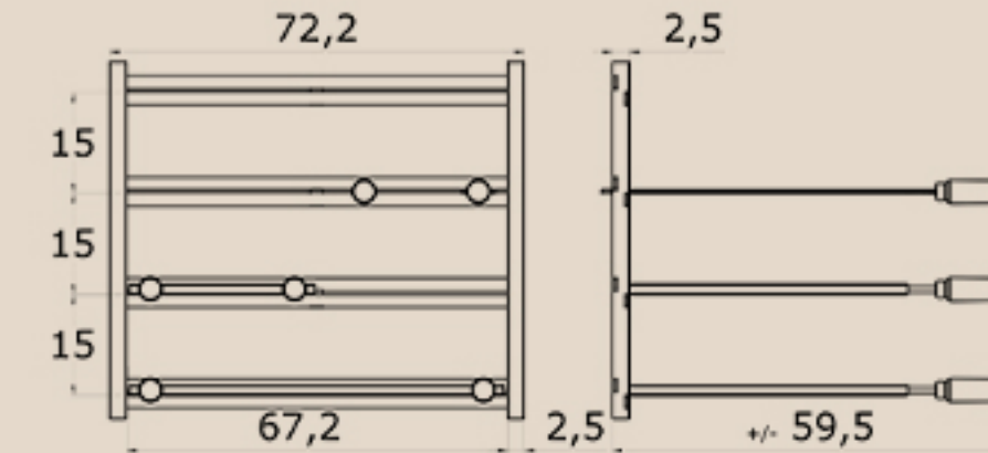
Grill Ossoboca Parede Modelo 3
