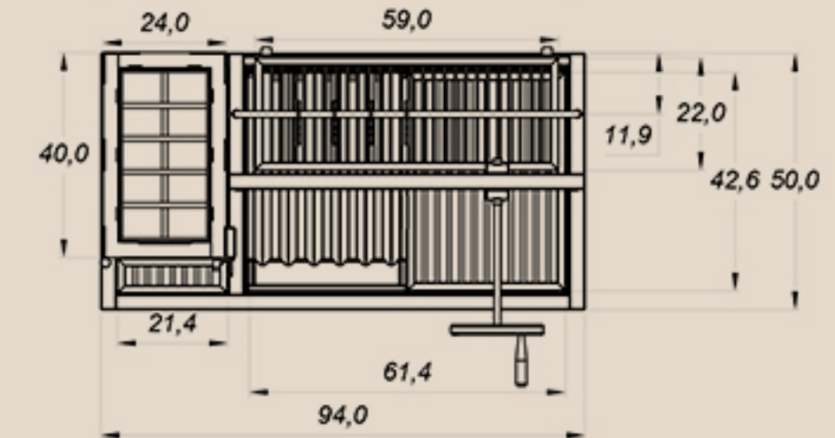
Bison Modelo 2 - 940x500 - VISTA SUPERIOR
