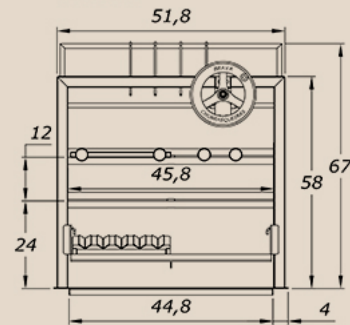
Elevation Grill Modelo 1
