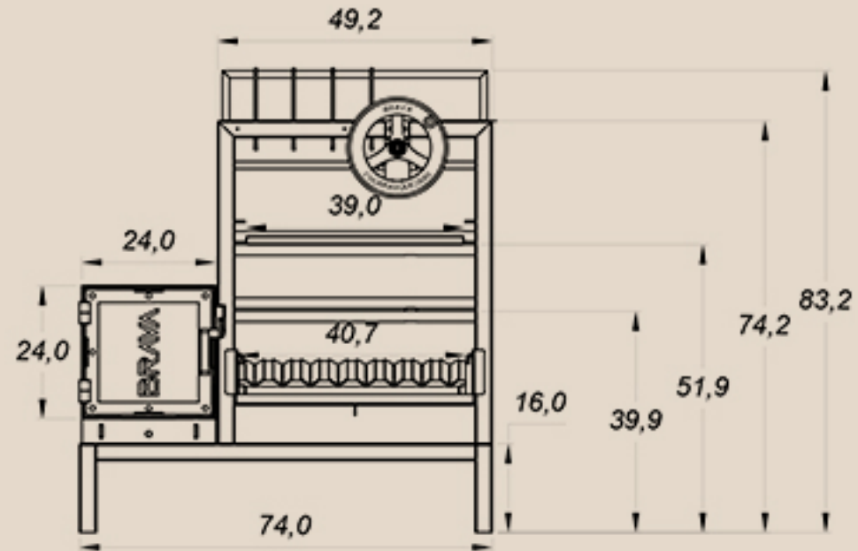
Bison Modelo 1 - 740x500 - VISTA FRONTAL
