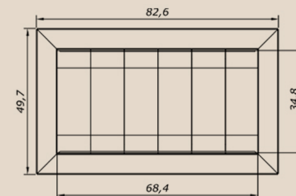
Braseiro Modelo 3 Corte Nicho: 77x44
