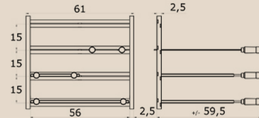
Grill Ossoboca Parede Modelo 2
