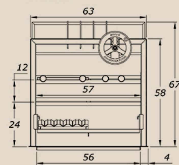
Elevation Grill Modelo 2
