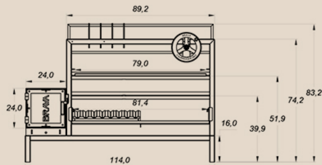
Bison Modelo 3 - 1140x500 - VISTA FRONTAL
