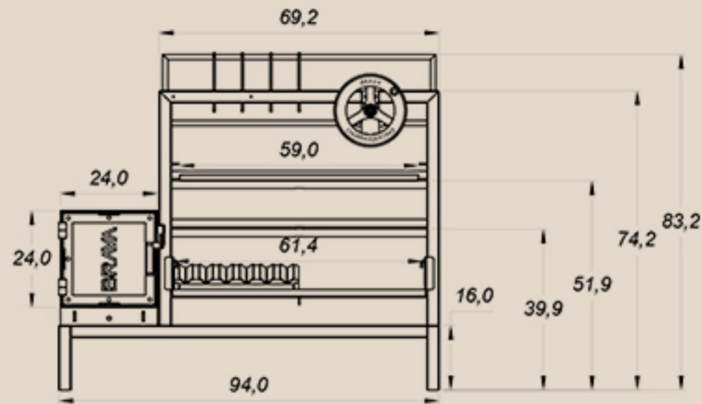
Bison Modelo 2 - 940x500 - VISTA FRONTAL
