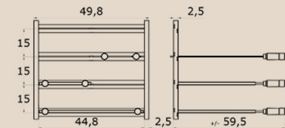
Grill Ossoboca Parede Modelo 1
