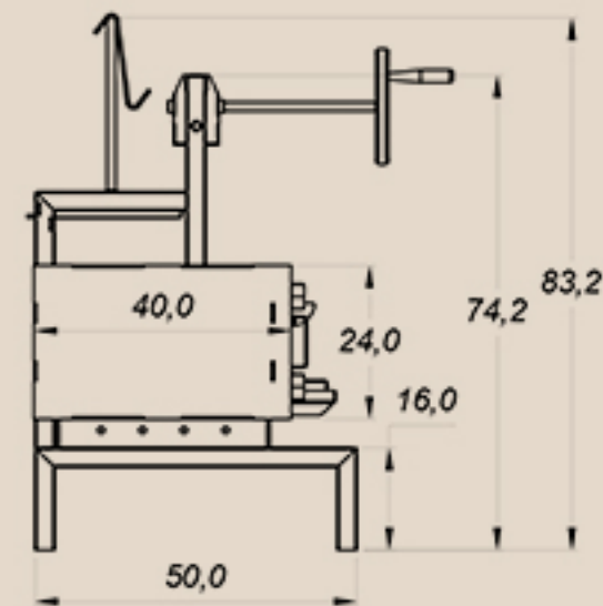
Bison Modelo 2 - 940x500 - VISTA LATERAL ESQUERDA
