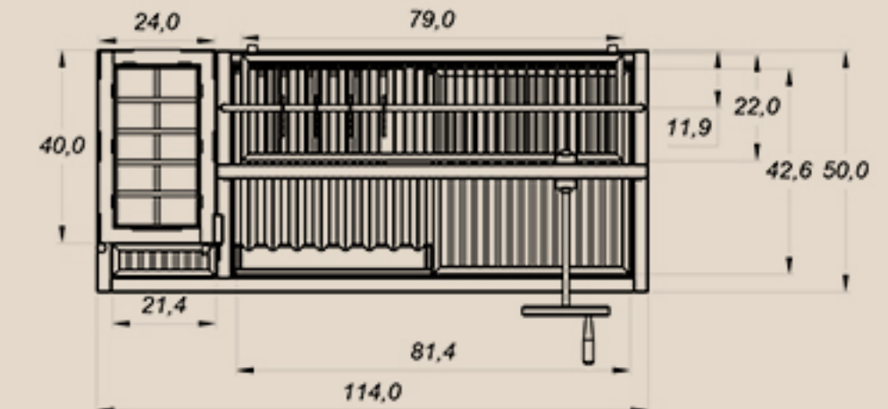
Bison Modelo 3 - 1140x500 - VISTA SUPERIOR
